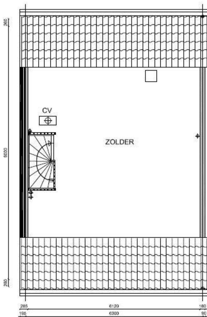
2e VERDIEPING
