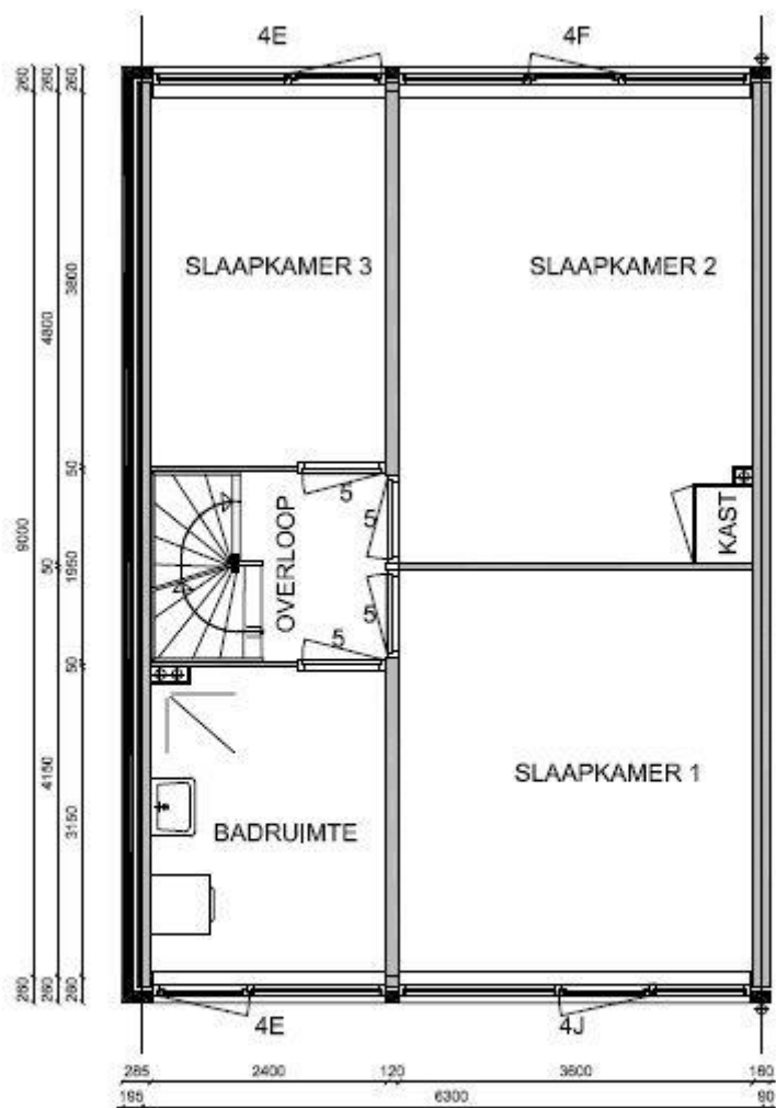
1e VERDIEPING
