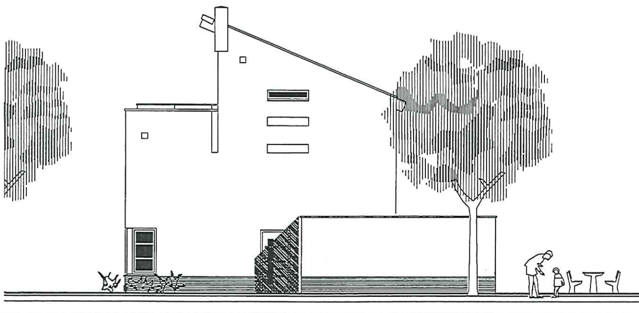
ZIJGEVEL ENTREE
