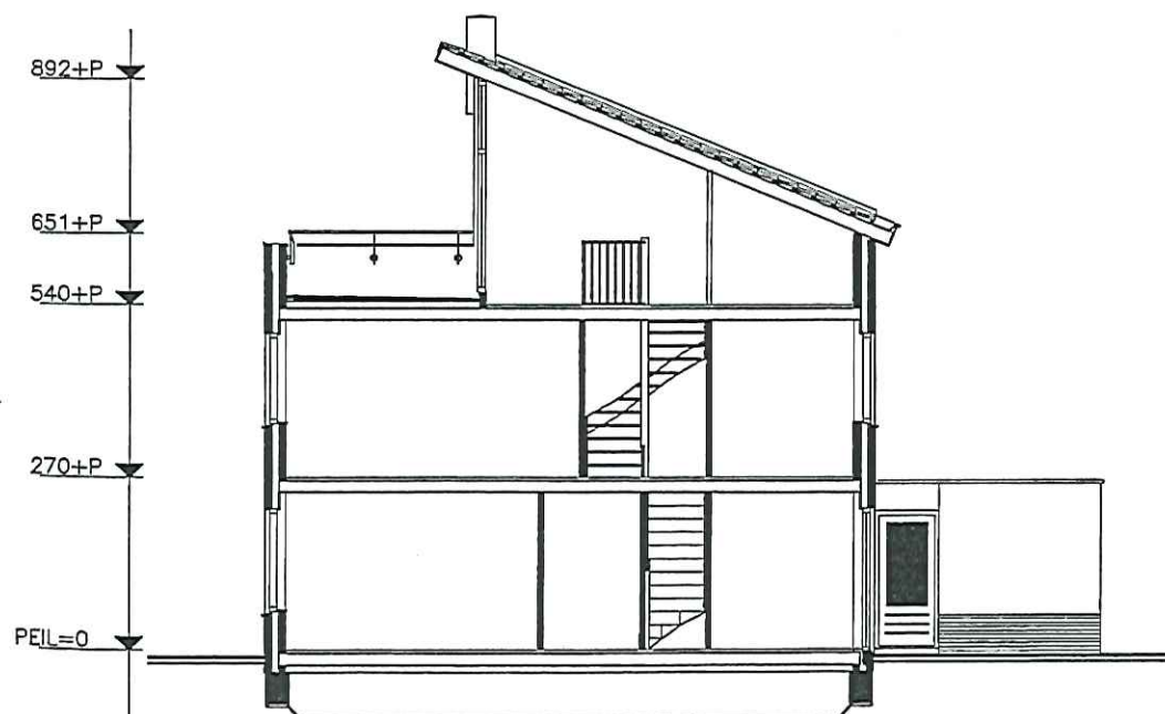
DOORSNEDE
